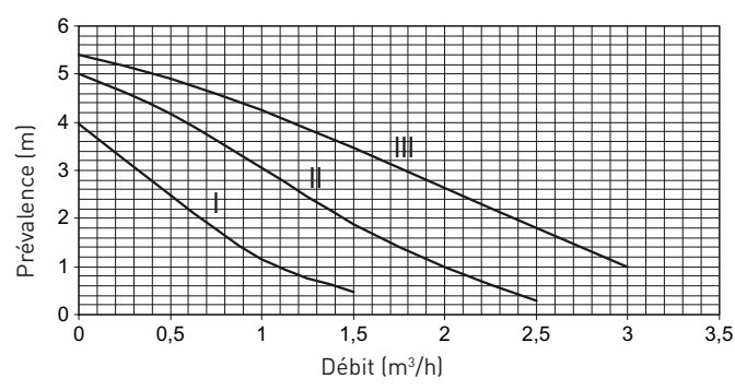
PRÉVALENCE POUR LES TROIS VITESSES DE LA POMPE SOLAIRE WILO ST 15/6 ECO
