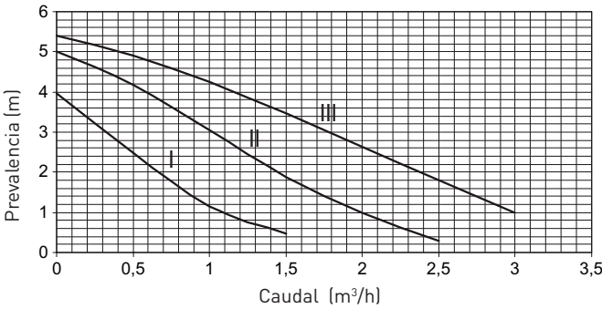
PREVALENCIA PARA LAS TRES VELOCIDADES DE LA BOMBA SOLAR WILO ST 15/6 ECO
